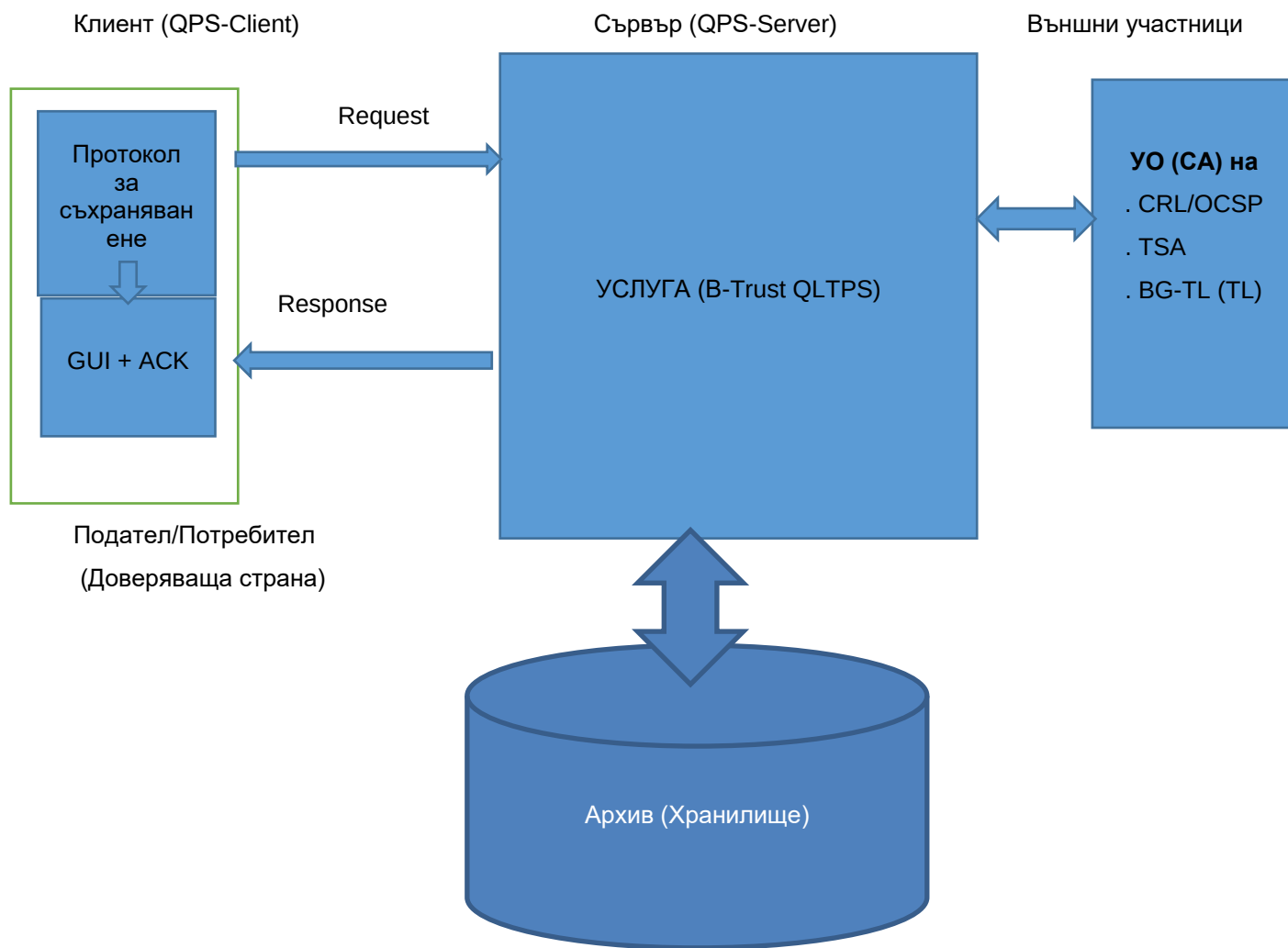
Фиг.1 Функционален модел на УСЛУГАТА
